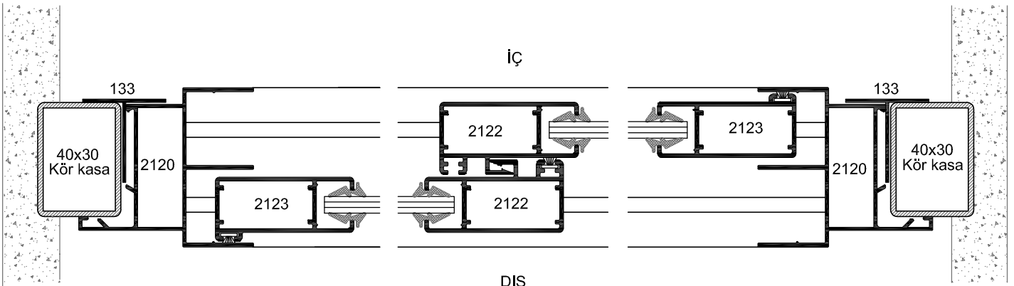
DETAY - 1
