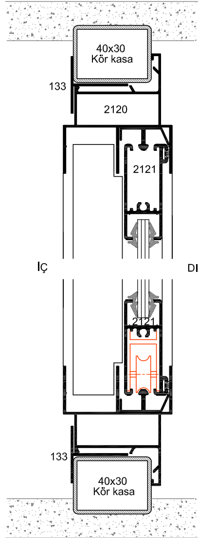
DETAY - 5
